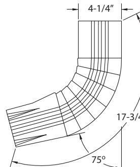
AAE245 A-Elbow
