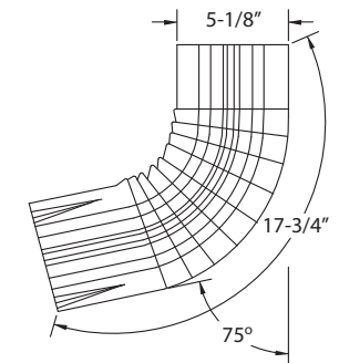
ABE245 B-Elbow
