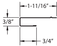
AJ38 - -
